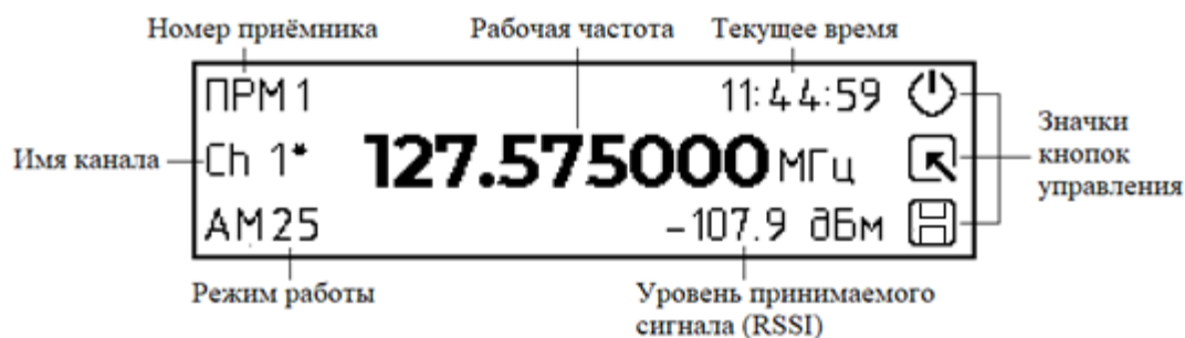
Рисунок 6 – Главный экран управления
