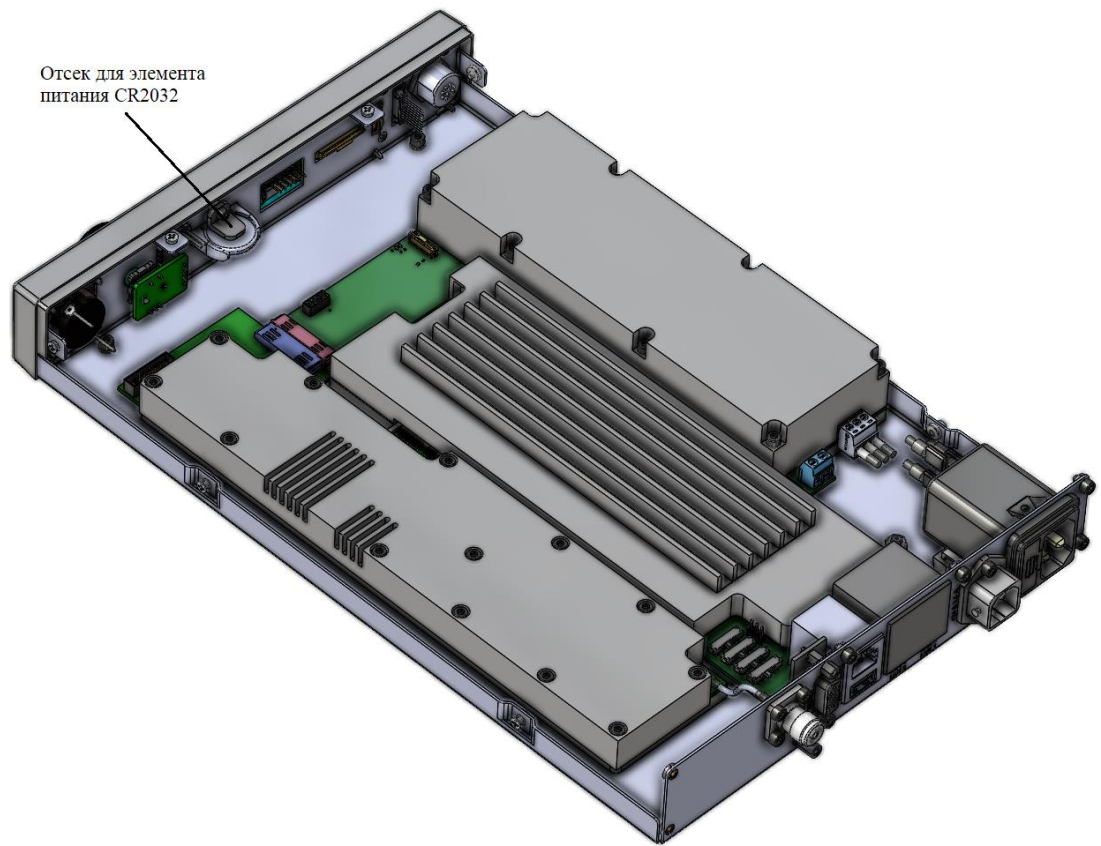
Рисунок В.1 – Расположение батарейного отсека
