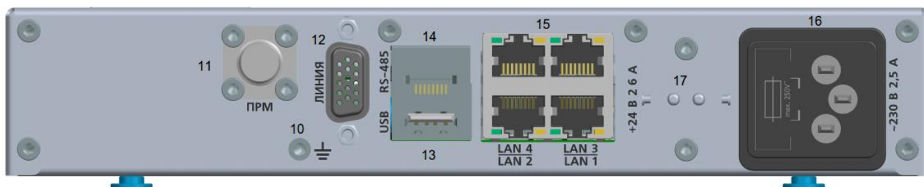
Рисунок 2 – Задняя панель Изделия
