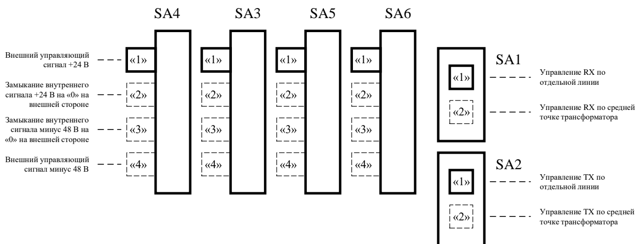
Рисунок Б.1 – Схема расположения движковых переключателей на модуле процессорном, задающих вид управления Изделием по НЧ-линии
