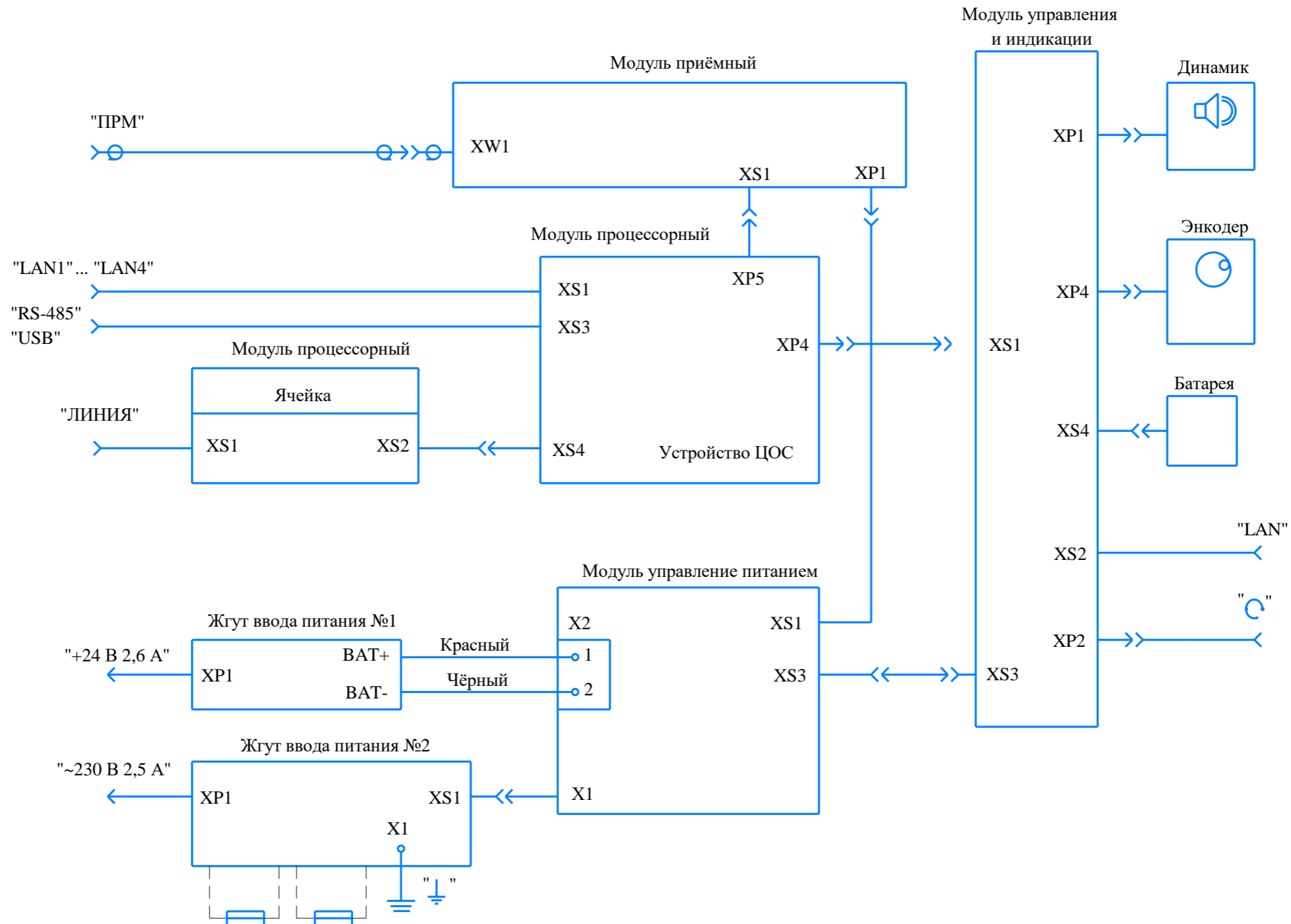
Рисунок 3 – Структурная схема Изделия
