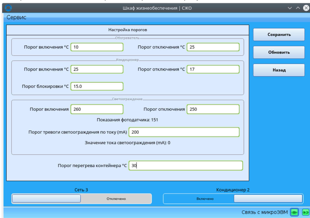
Рисунок 16. Вид окна с настройками порогов.
